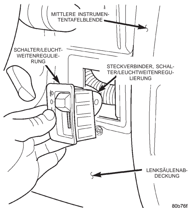
Abb. 2 Steckverbinder des Schalters/Leuchtweitenregulierung
