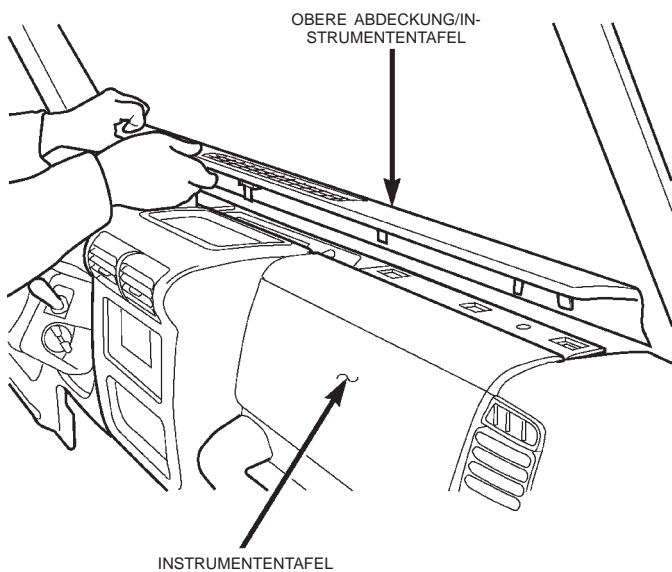
Abb. 3 Obere Abdeckung der Instrumententafel
