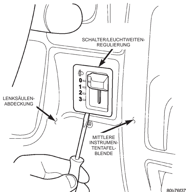
Abb. 1 Schalter/Leuchtweitenregulierung
