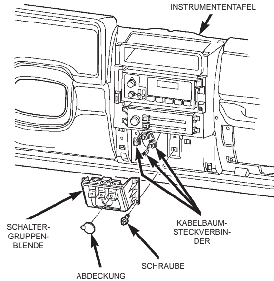
Abb. 6 Schaltergruppenblende
