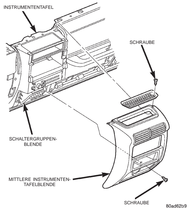
Abb. 4 Untere Befestigungsschraube der mittleren Blende
