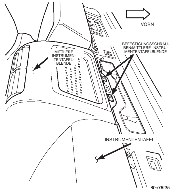
Abb. 5 Befestigungsschrauben der mittleren Instrumententafelblende
